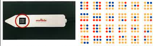
<9電極を用いたECセンサ計測パターン例>
